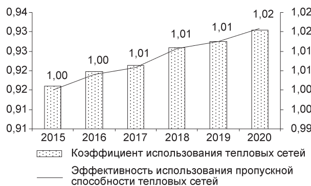
Рис. 10. Показатели эффективности использования пропускной способности тепловых сетей Республики Беларусь, 2015–2020 гг.
